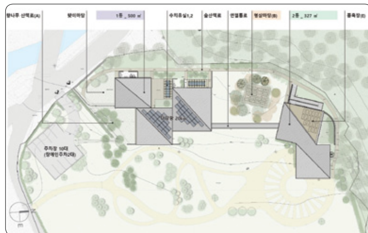
녹색복지센터 배치도
